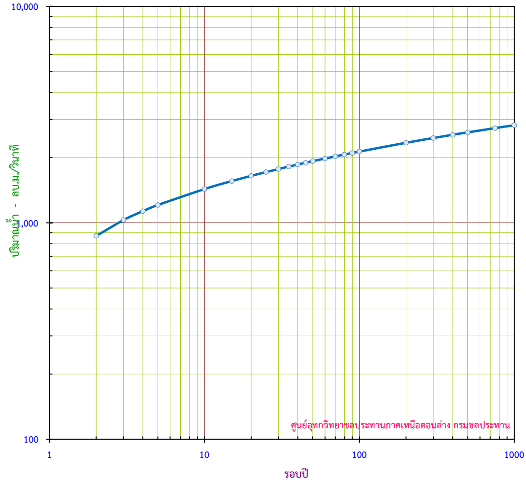
กราฟแสดง ปริมาณน้ำสูงสุดรายปี ขนาดรอบปีต่างๆ สถานี N.74 บ.บางกระพุ่ม อ.บางกระพุ่ม จ.พิษณุโลก
